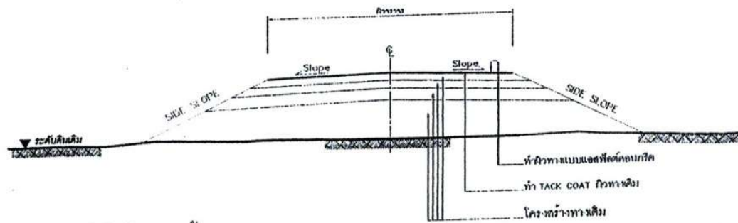
รูปตัดโค้งสร้างทาง 1
