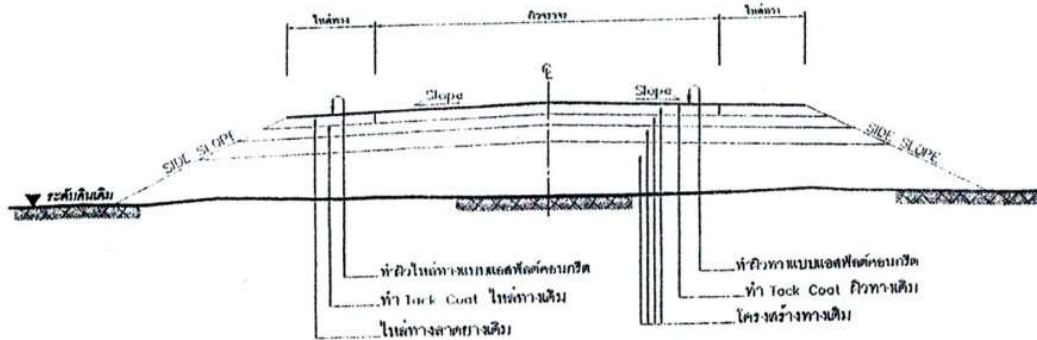
รูปตัดโค้งสร้างทาง 2
